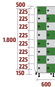
FZ-30/2 COD: 53171 107kg · 0,54m 3
