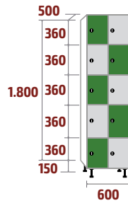
FP-30/2 COD: 53151 91kg · 0,54m 3
