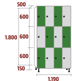
FM-30/4 COD: 53133 148kg · 1,07m 3
