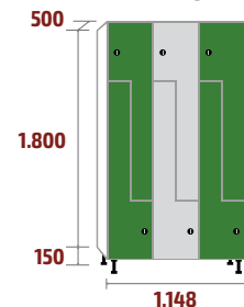
FL-40/3 COD: 53185 150kg · 1,06m 3
