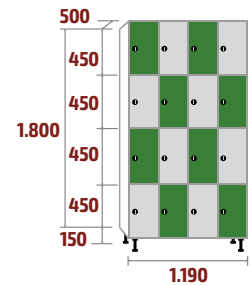
FC-30/4 COD: 53143 158kg · 1,07m 3
