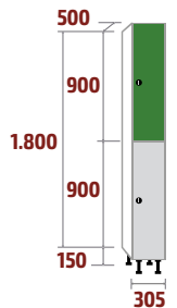
FT-30/1 COD: 53011 44,1kg · 0,27m 3
