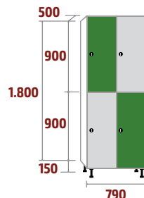
FT-40/2 COD: 53123 85,85kg · 0,71m 3
